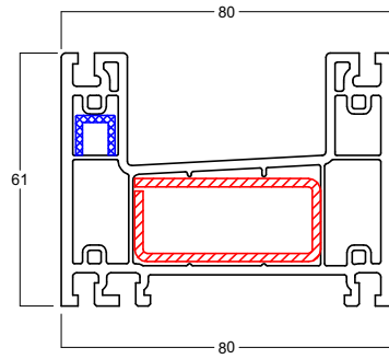
61mm Outer Frame Art No: 6052 Reinf V107
